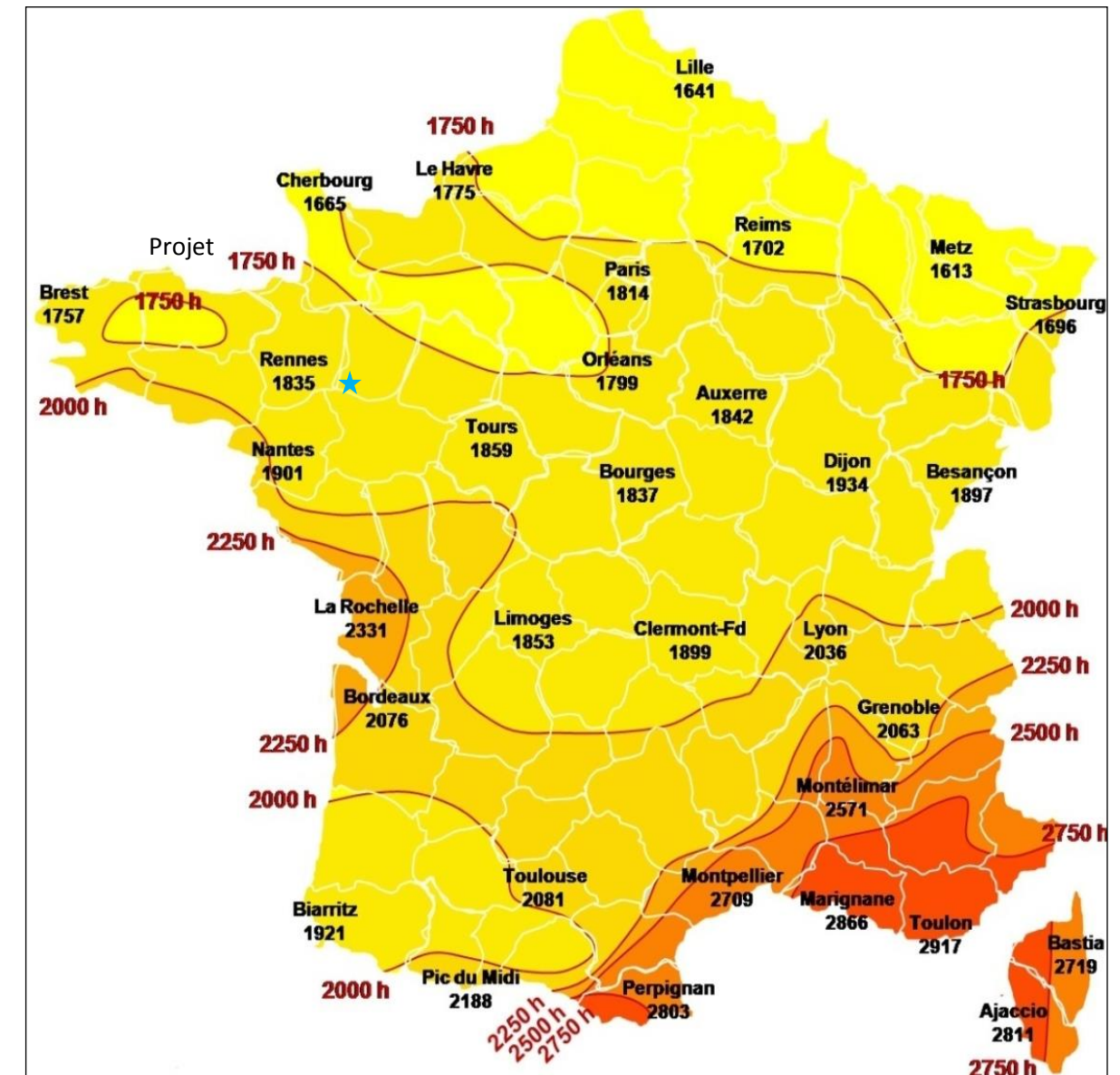
Figure 17 : Ensoleillement en France, en nombre d'heures/an
