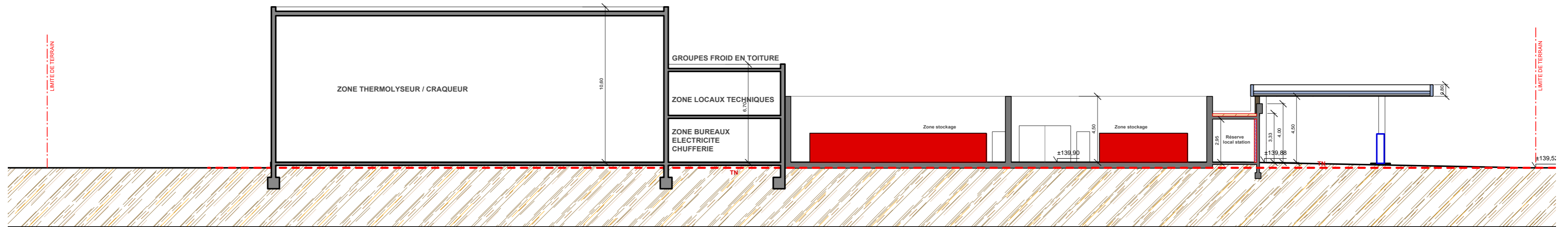
COUPE CC ETAT PROJETE Ech. 1/200
